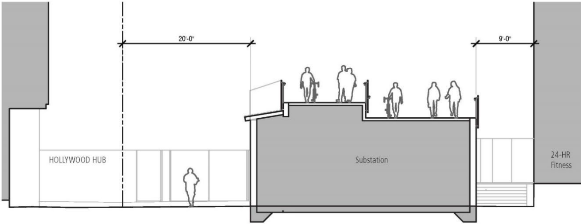
3 STRAMP SECTION - SUBSTATION Scale: 1/8" = 1'-0"
