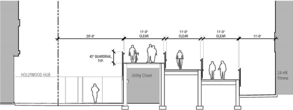
2 STRAMP SECTION - UTILITY CLOSET Scale: 1/8" = 1'-0"
